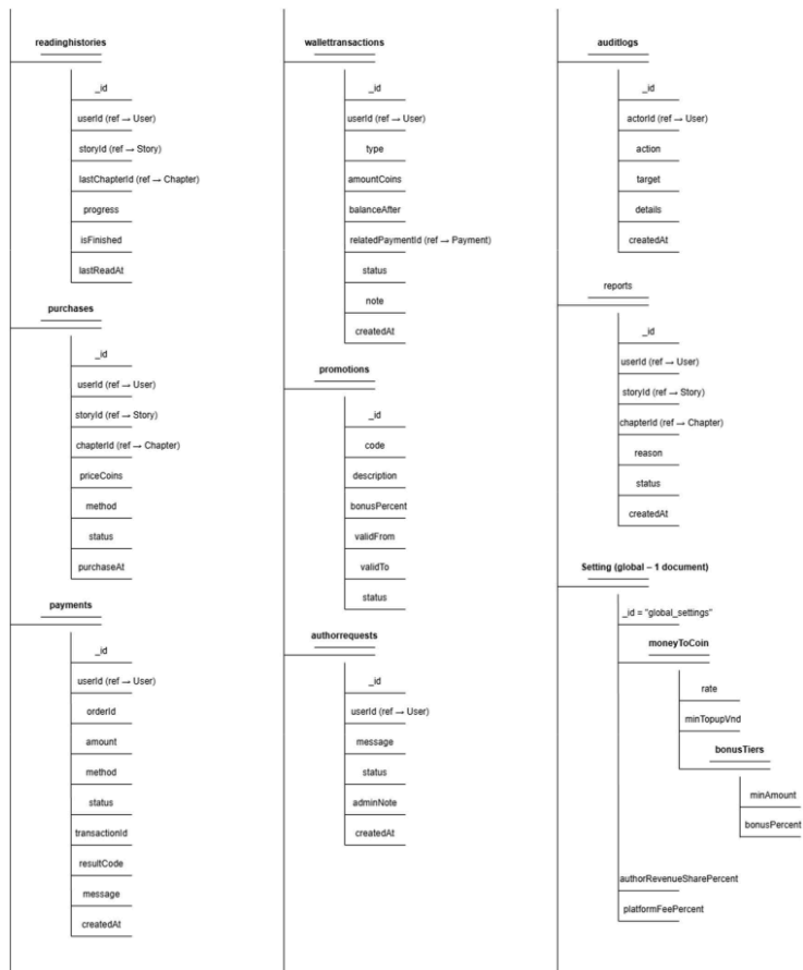
Hình 17: Data Structure MongoDB - Phần 2
