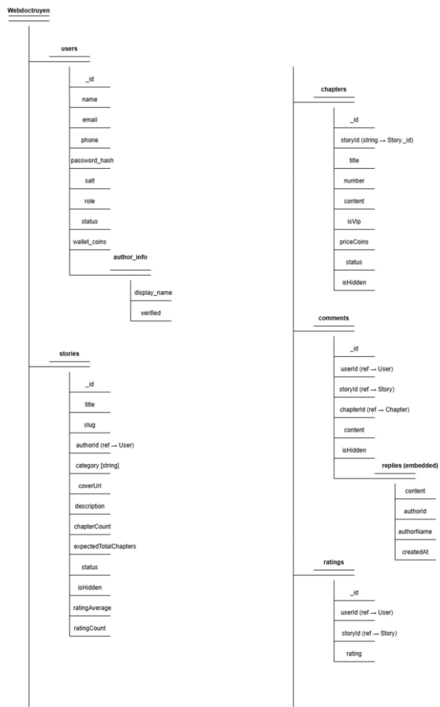
Hình 16: Data Structure MongoDB – Phần 1
