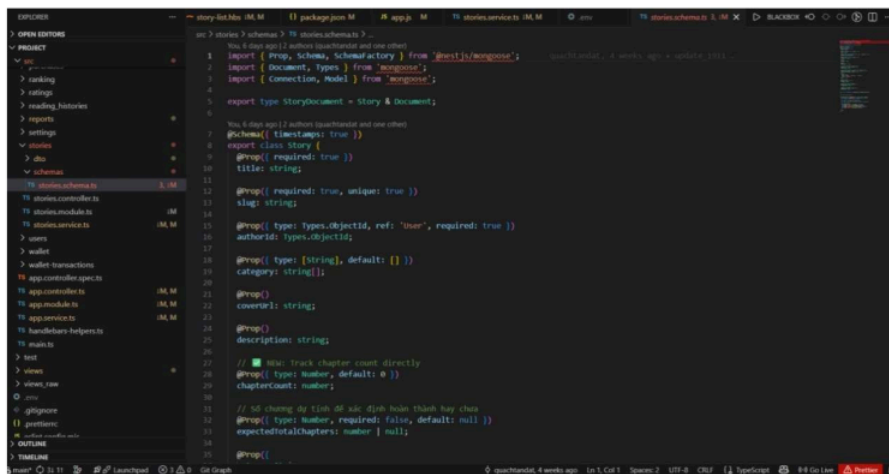
Hình: File schema
