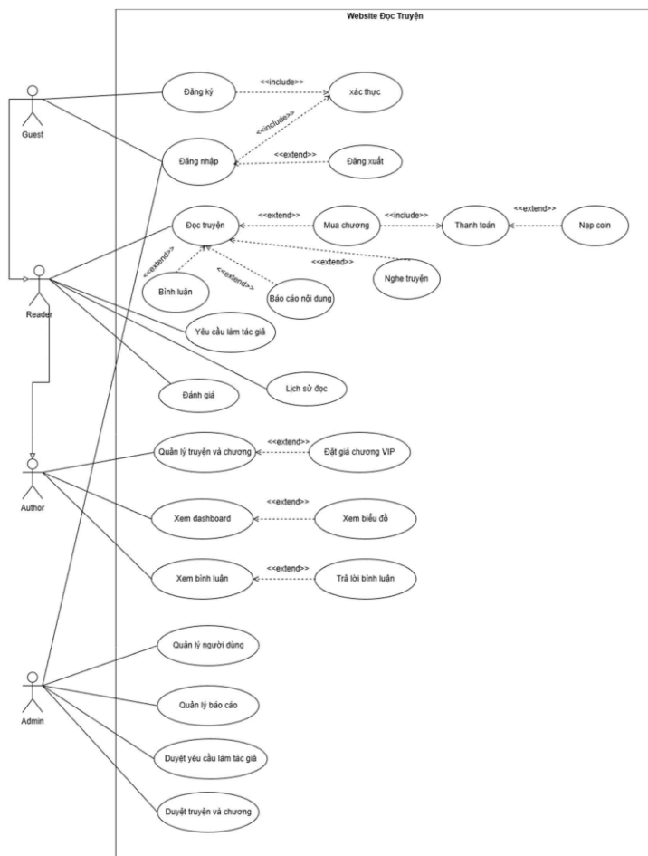
Hình 5: Use Case Diagram
